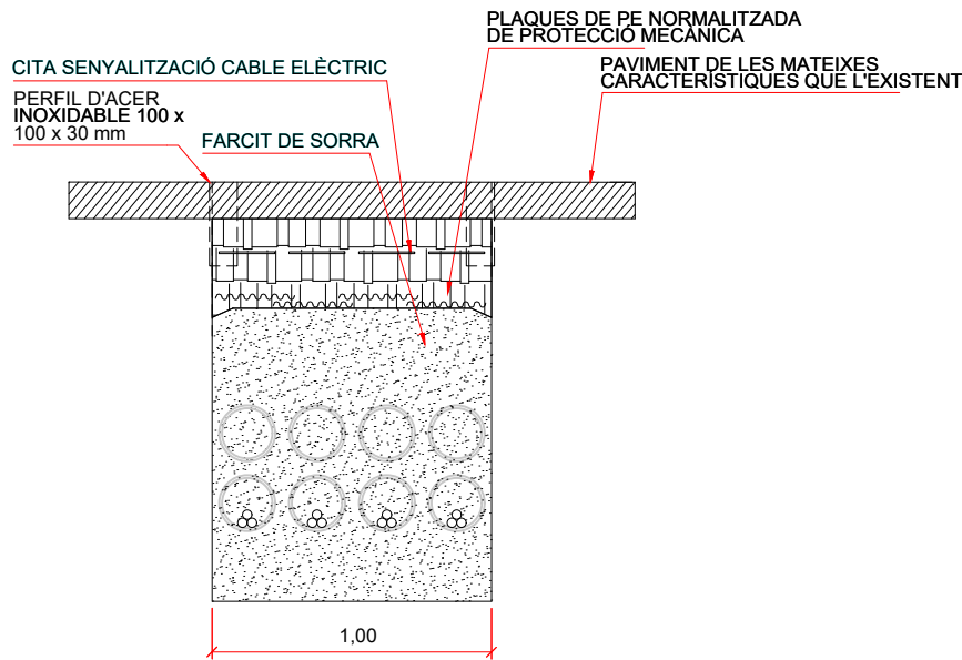
SECCIÓ B-B'
