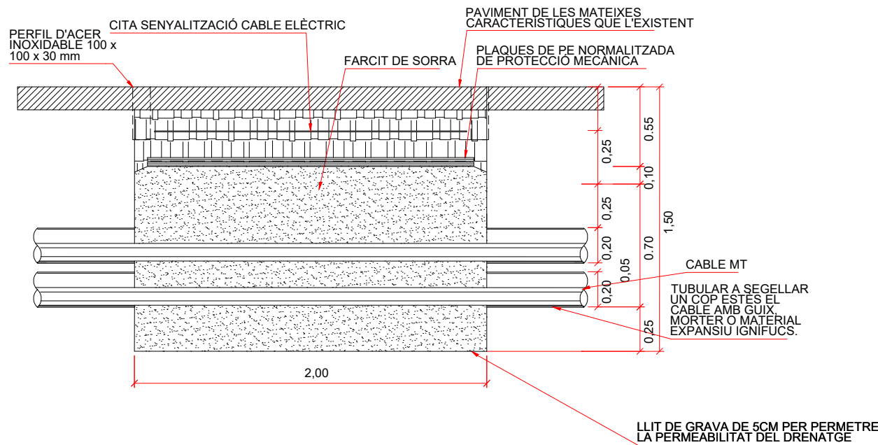
SECCIÓ A-A'
