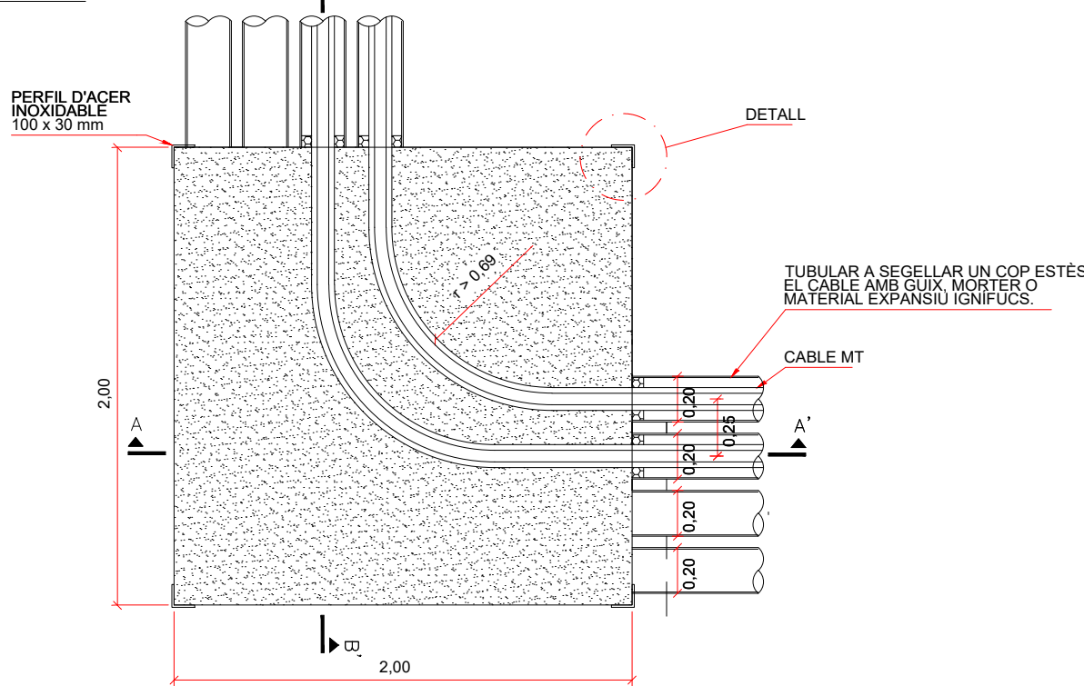
PLANTA
