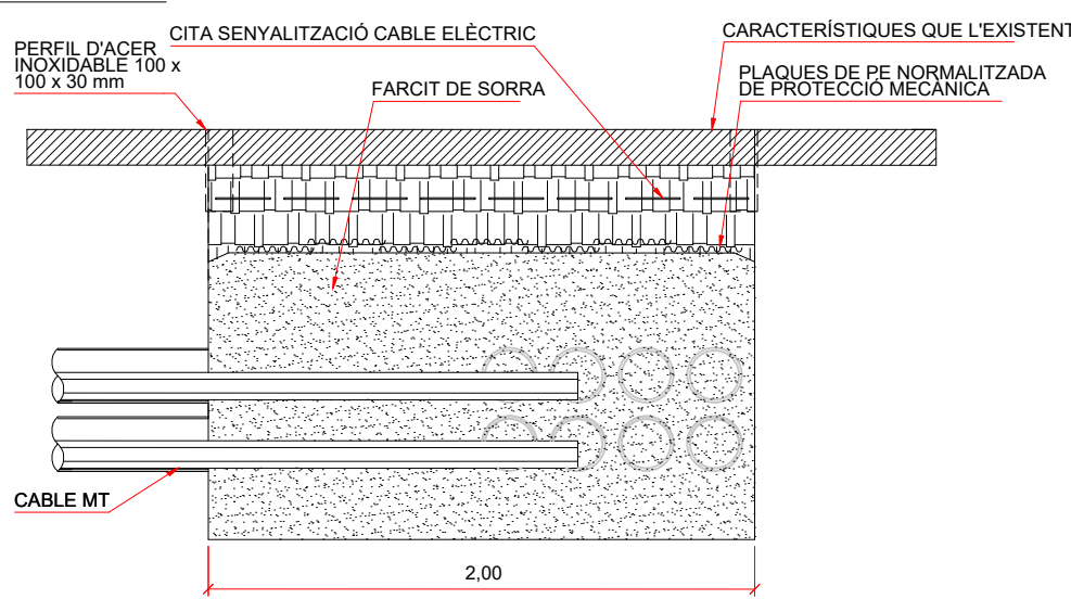
SECCIÓ B-B'
